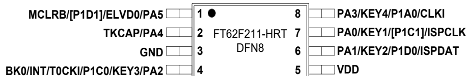
图 1-5 DFN8 3
